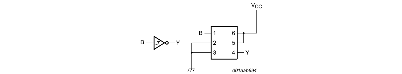
Fig. 12. Inverter
