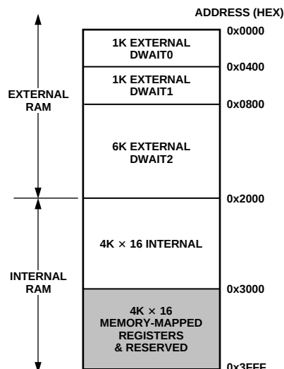
Figure 7. ADSP-2165/ADSP-2166 Data Memory Map
