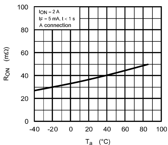
Fig. 12.1.5 R_{ON} - T_a
