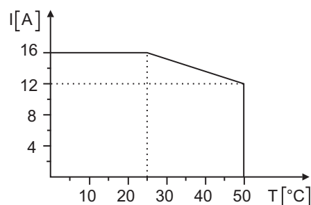
Deratingkurve (Im angereiztem Zustand)
