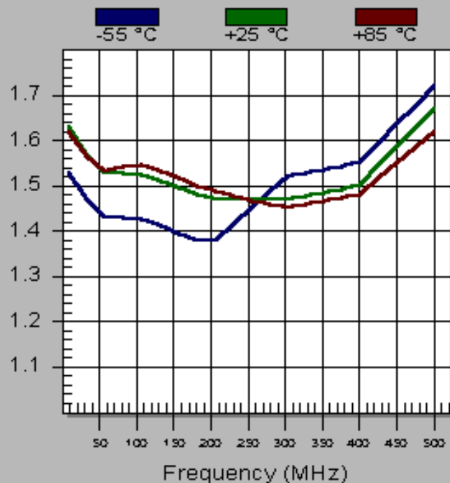
TM6507 Output VSWR
