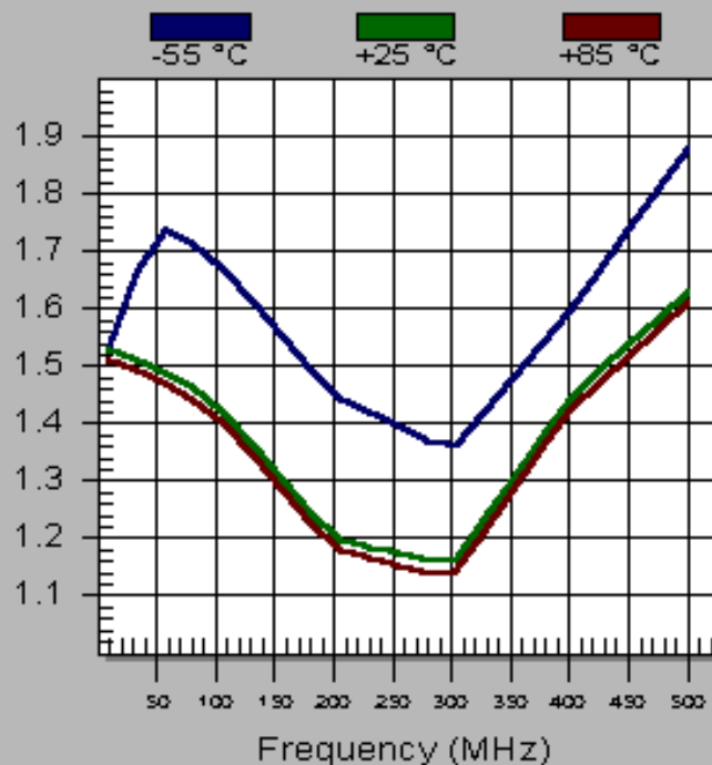
TM6507 Input VSWR
