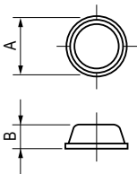
TM-166-12・12W
