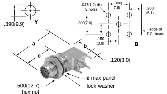
PCB Angle Bulkhead Receptacle (J) 81-119-1007
