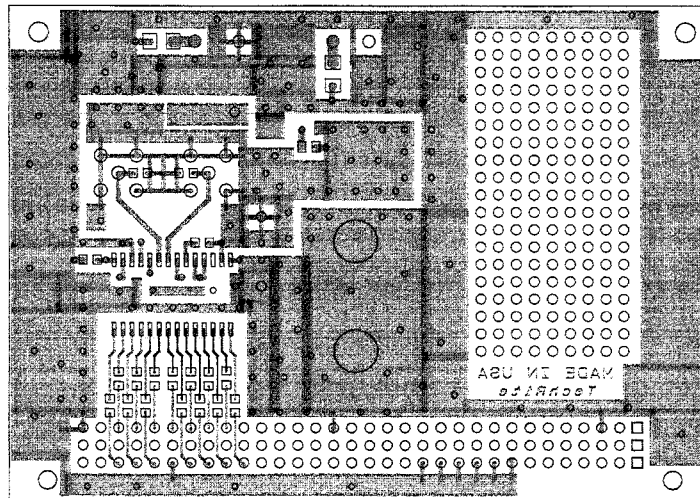
FIGURE 19E. LAYER 4
