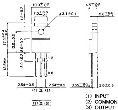
TO220FP
