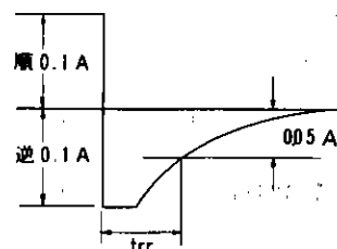
注1 逆回復時間測定波形
