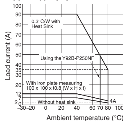
G3NA-490B-UTU-2
