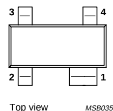
Fig.2 SOT143R.
