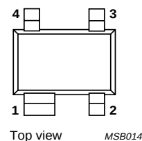
Fig.1 SOT143B.
