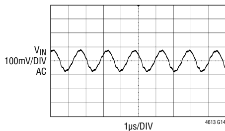
Input Ripple
