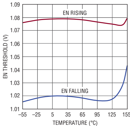
EN Thresholds
