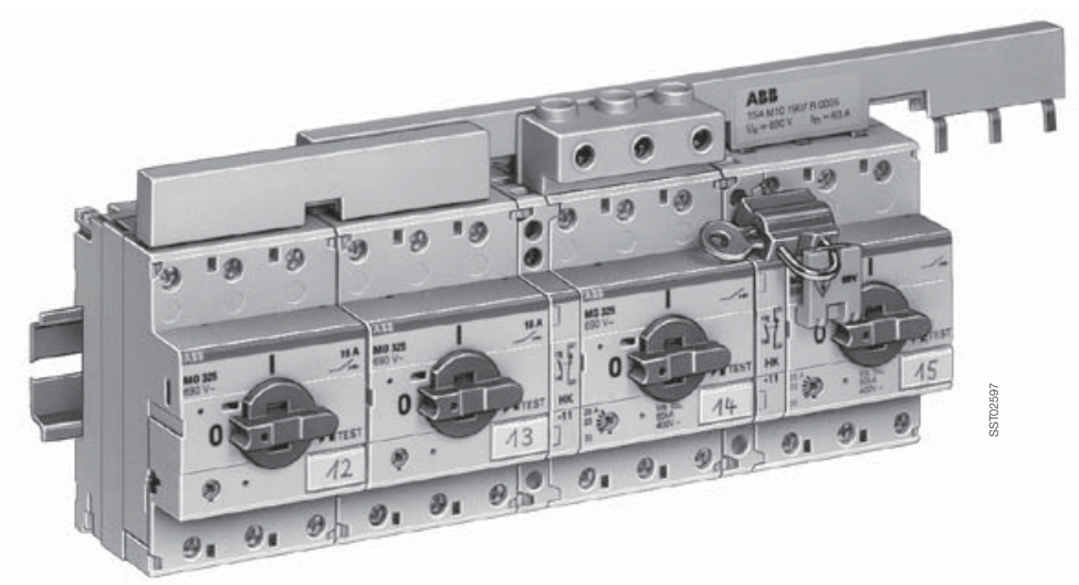
MS 325 mit Hilfsschalter HK querverdrahtet mit Phasenschiene und Einspeiseblock
