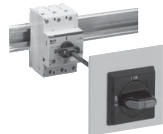
Schaltschrankeinbau
