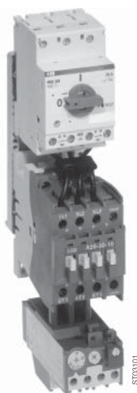
MO 325 mit Schütz A 26 sowie thermischen Überstromrelais TA 25 DU
