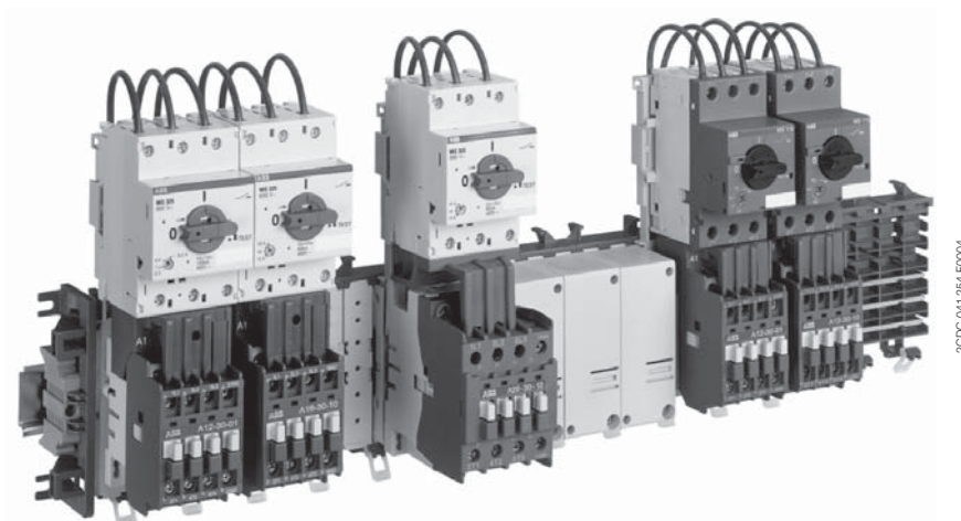
Starter-Kombinationen mit Kombimodulen auf Stecksocket-Schienensystem SMISSLINE bis 100 A, max. Einspeisequerschnitt: 95 mm 2 ①
