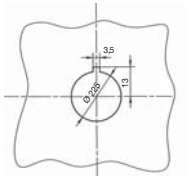
Bohrplan
