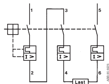
Motorschuttschalter zum Schalten von Gleichstrom und Einphasen-Wechselstrom
