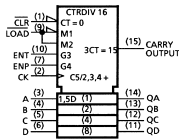
TC74ACT161
