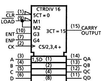
TC74ACT163
