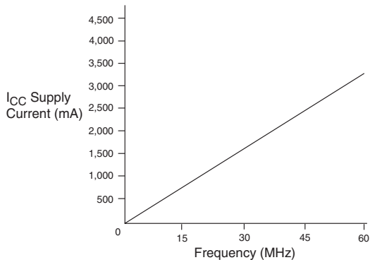
EPF10K100
