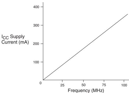
EPF10K30A
