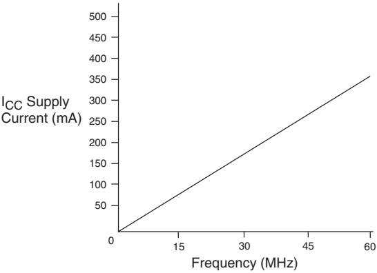
EPF10K30
