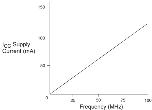
EPF10K10A
