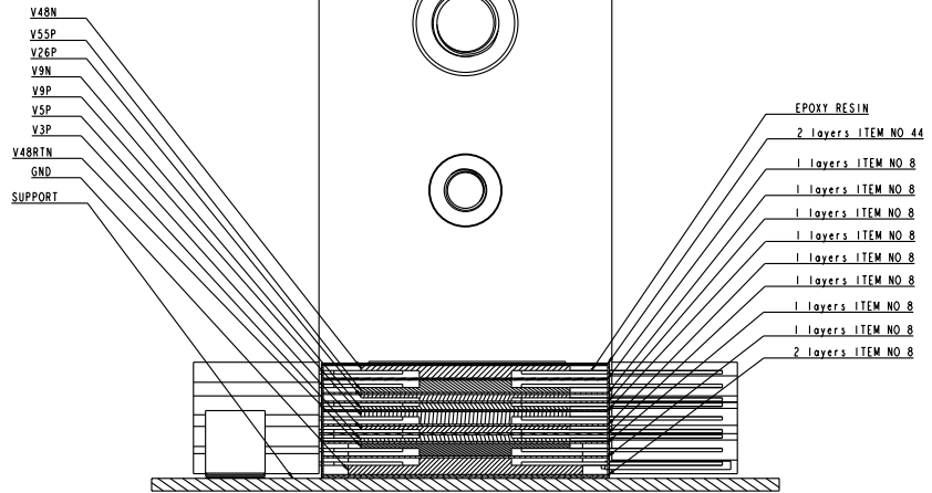
SECTION A-A SCALE 1.000
