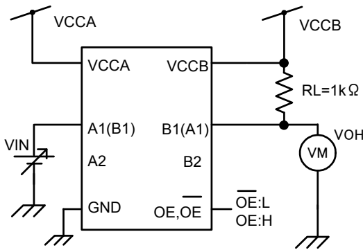
図 7 測定回路
