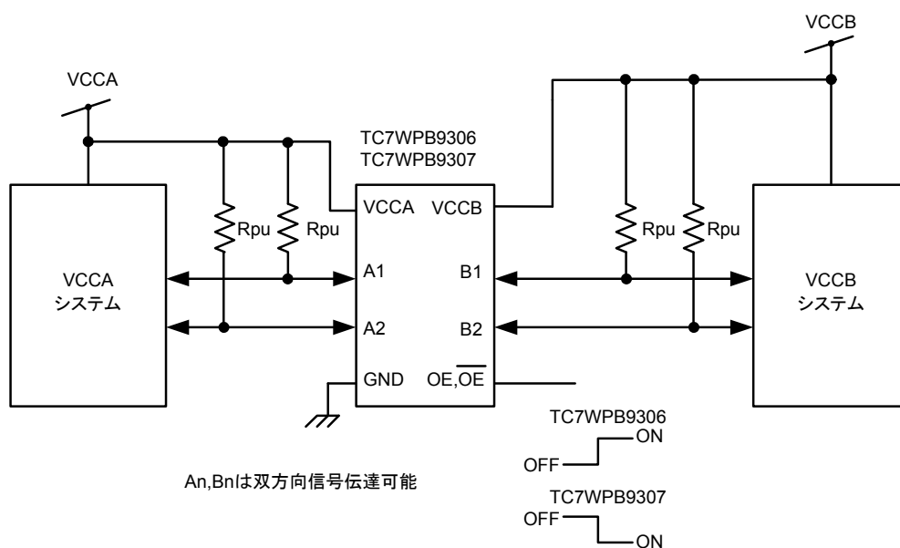
図1 応用回路図
