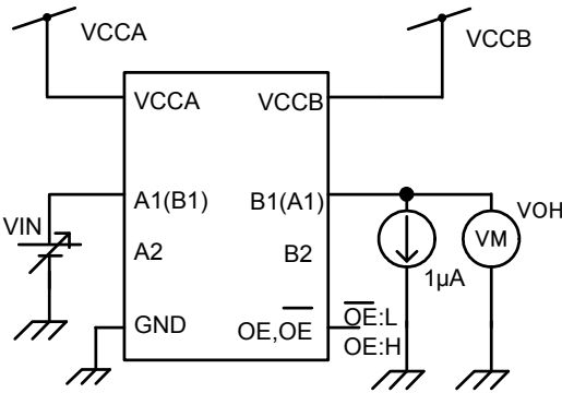
図 9 測定回路
