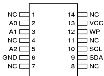
14-Pin SOIC
