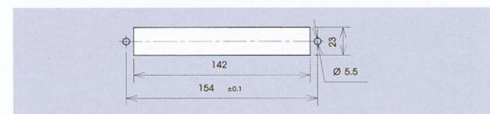
Montageöffnung · Mounting Opening
