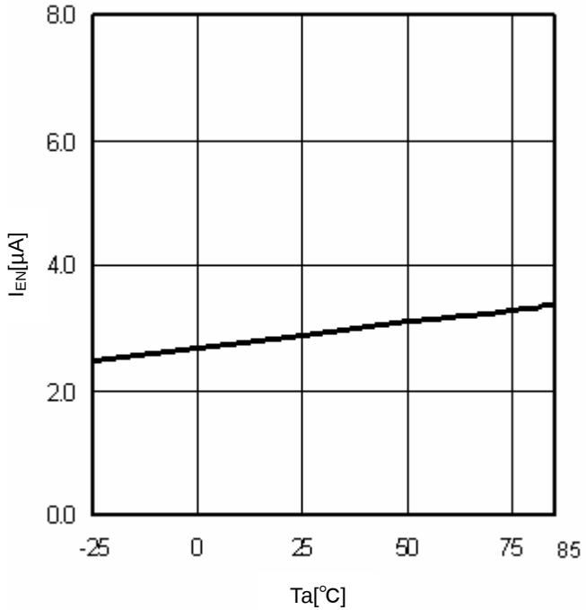
Fig.12 T_a - I_{EN}
