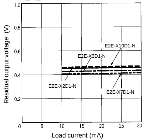
E2E-X□D□
