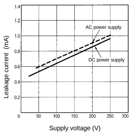
E2E-X□T1
