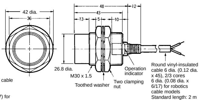
Fig. 16 : E2E-X20MD□/E2E-X18ME□/F□ E2E-X18MY□
