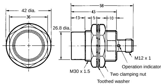
Fig. 26 : E2E-X20MD□-M1G/E2E-X18ME□-M1/F□-M1 E2E-X18MY□-M1
