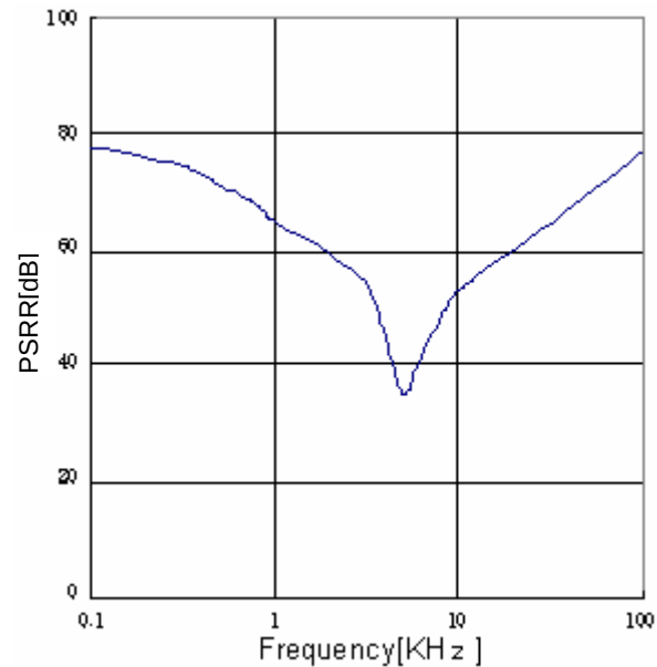
Figure 32. PSRR(Io=0mA)
