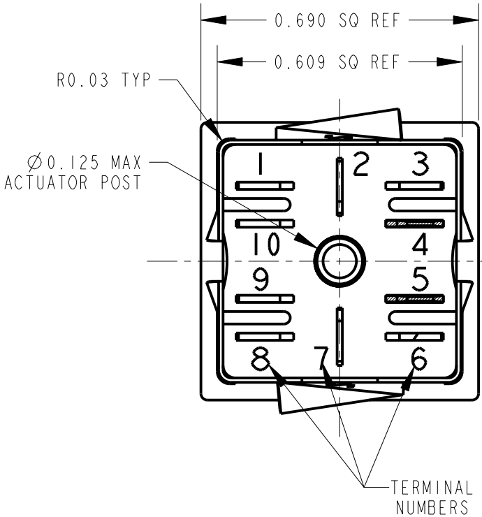
SCHEMATIC 1-A
