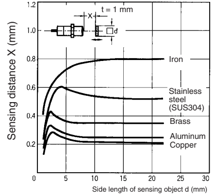
E2E-CR8□□
