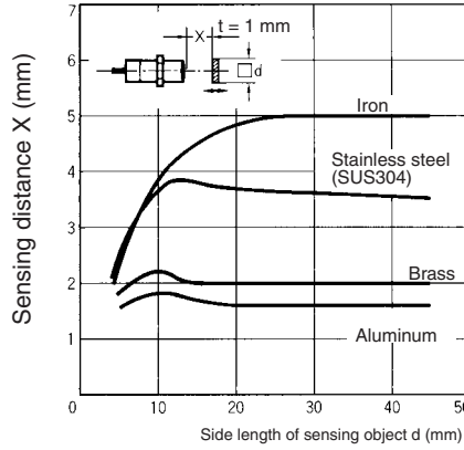
E2E-CR6□□
