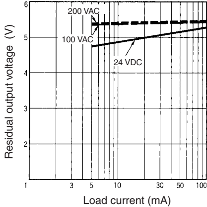
E2E-X□T1
