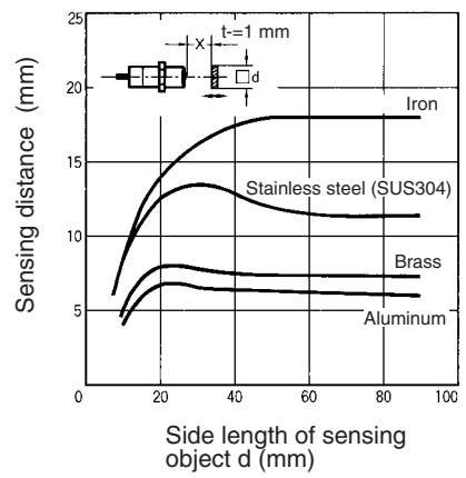
E2E2-X18MC/B E2E2-X18MY
