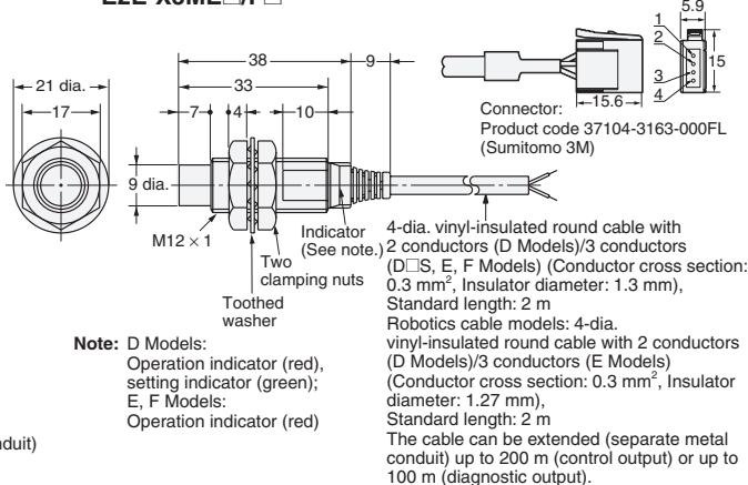
Fig. 10: E2E-X8MD□ E2E-X5ME□/F□
