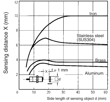
E2E-CR8□□
