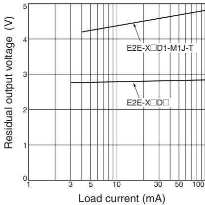
E2E-X□D□
