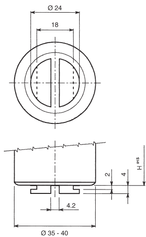
Fissaggio rapido a slitta solo per dia 30-35-40 mm (su richiesta) Quick mounting slider for dia 30-35-40 mm only (on request)
