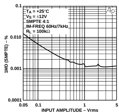
Figure 10. SMPTE IM vs. Amplitude V_{rms}
