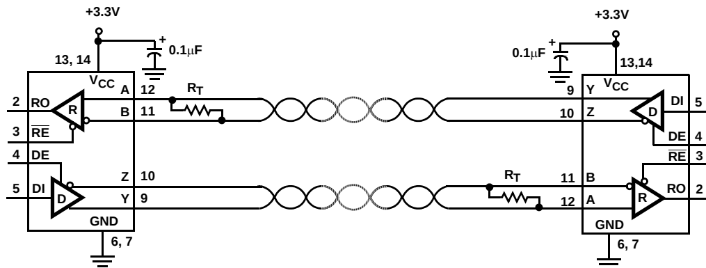
ISL83491
