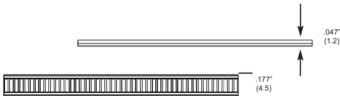
Strap ATS3080
