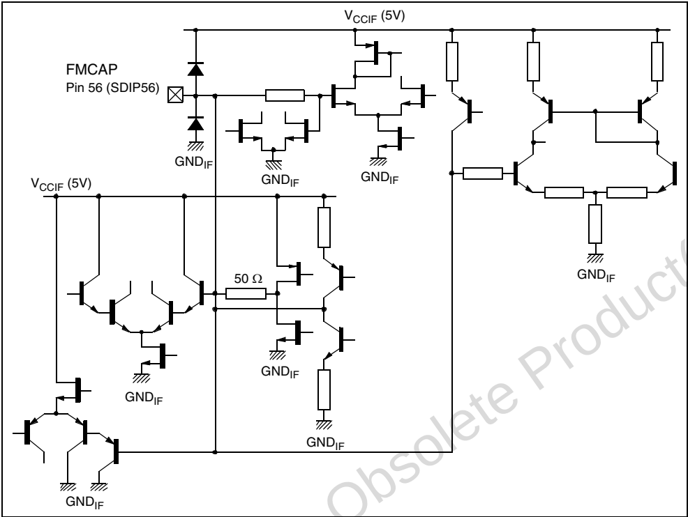
Figure 26. IF Inputs
