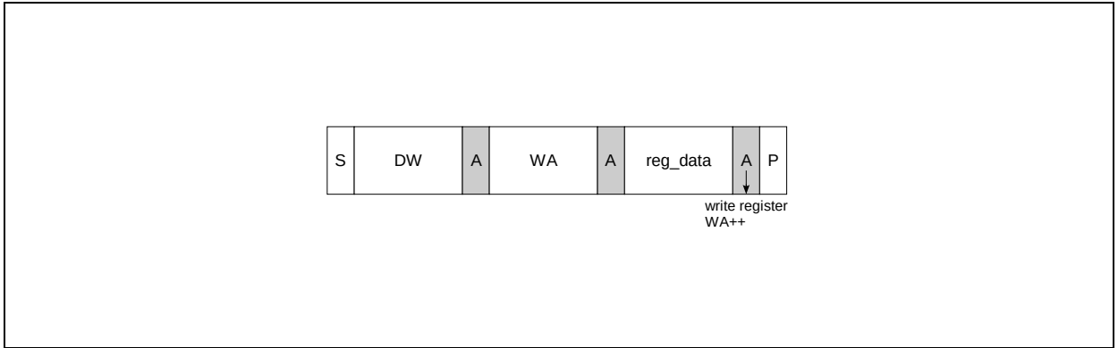
Figure 21. Byte Write
