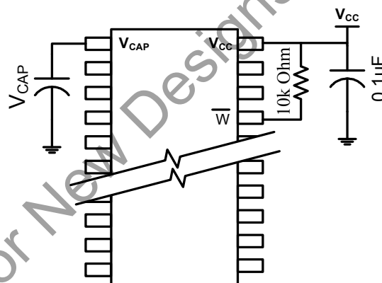
Figure 15. AutoStore Mode
