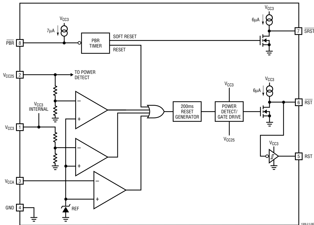
LTC1326-2.5
