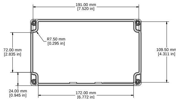
LID - INSIDE
