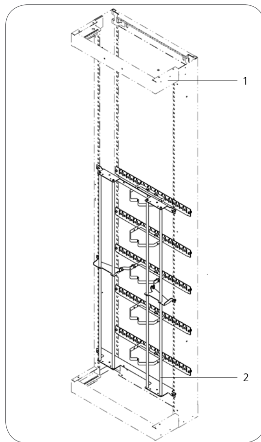
1 VtS-Tragegestell
