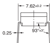
Flat Actuator
