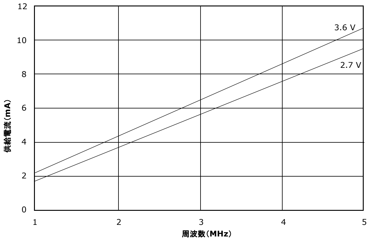
図 10. 標準 I_{CCI} と周波数
