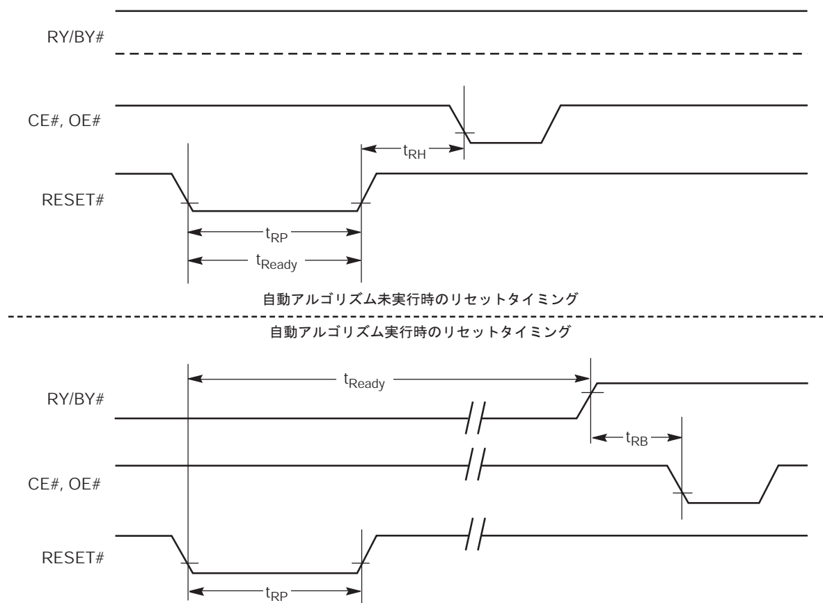
図 14. リセットタイミング
