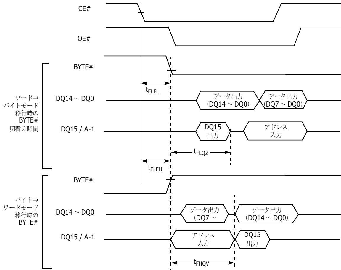
図 15. リード動作時の \text{BYTE}\# タイミング
