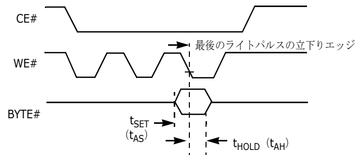
図 16. ライト動作時の \text{BYTE}\# タイミング
