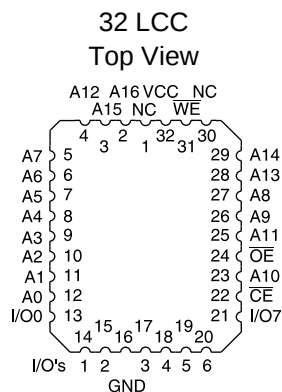
NC 1 32 VCC A16 2 31 WE A15 3 30 NC A12 4 29 A14 A7 5 28 A13 A6 6 27 A8 A5 7 26 A9 A4 8 25 A11 A3 9 24 \overline{OE} A2 10 23 A10 A1 11 22 \overline{CE} A0 12 21 I/O7 I/O0 13 20 I/O6 I/O1 14 19 I/O5 I/O2 15 18 I/O4 GND 16 17 I/O3
