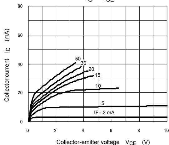
I_C - V_{CE}
