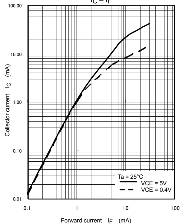
I_C - I_F
