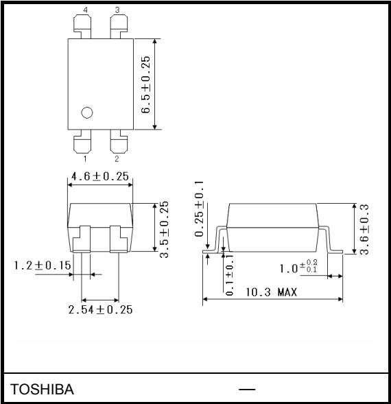
TLP781(LF6)
