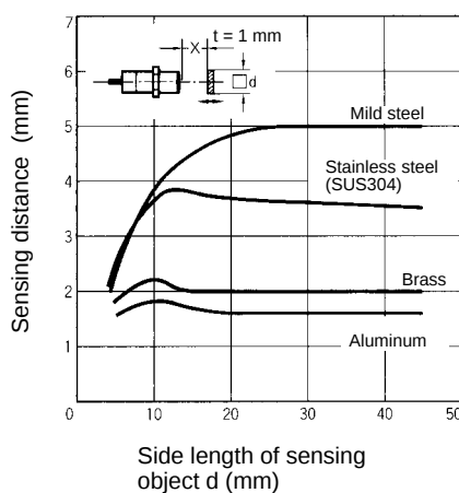
E2E-X5ME□/F□ E2E-X5MY□
