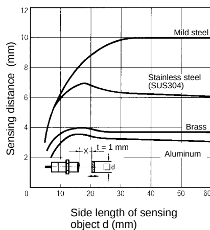
E2E-X10ME□/F□ E2E-X10MY□
