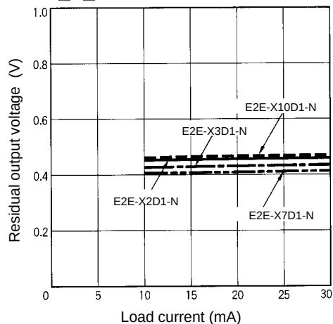
E2E-X□D□
