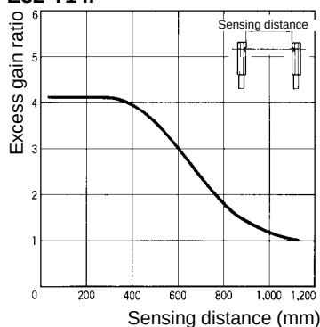
E32-T14F
