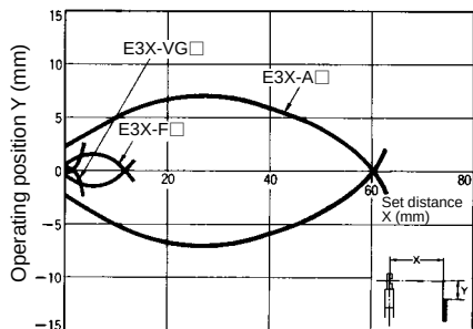
E32-D14L
