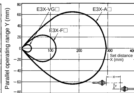
E32-T11
