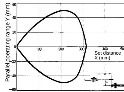
E32-T21L
