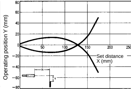
E32-D32L
