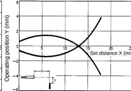
E32-D33
