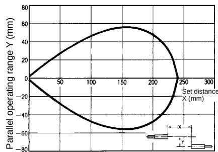
E32-T22
