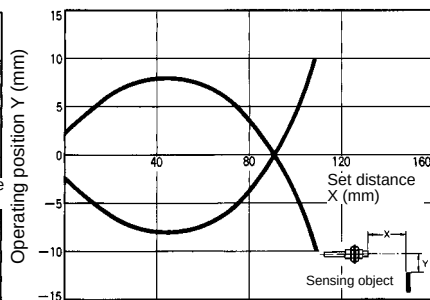
E32-D21L
