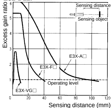
E32-D12F
