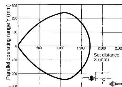
E32-T11L
