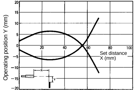
E32-D32
