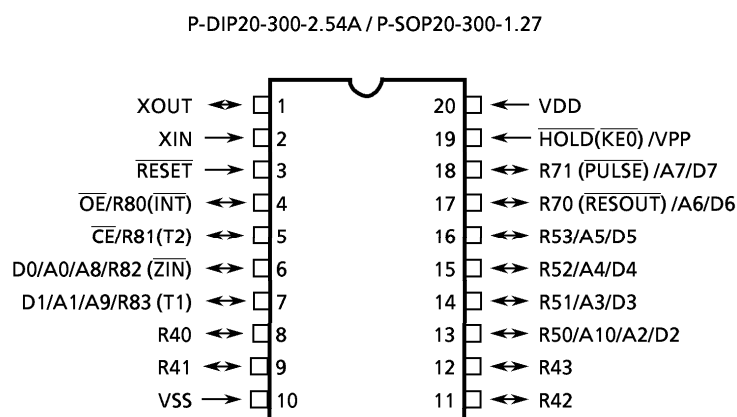
P-SOP20-300-1.27
