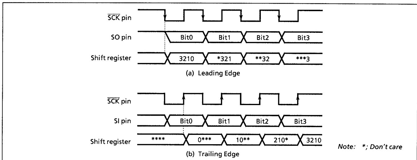
Figure 2-35. Shift Edge
