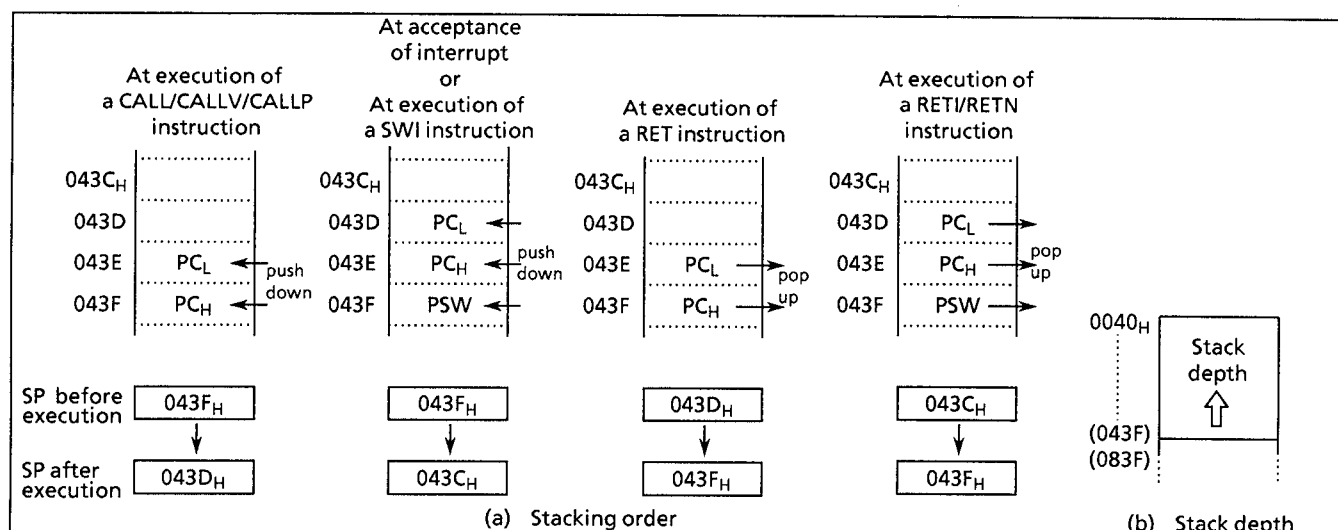
Figure 1-8. Stack
