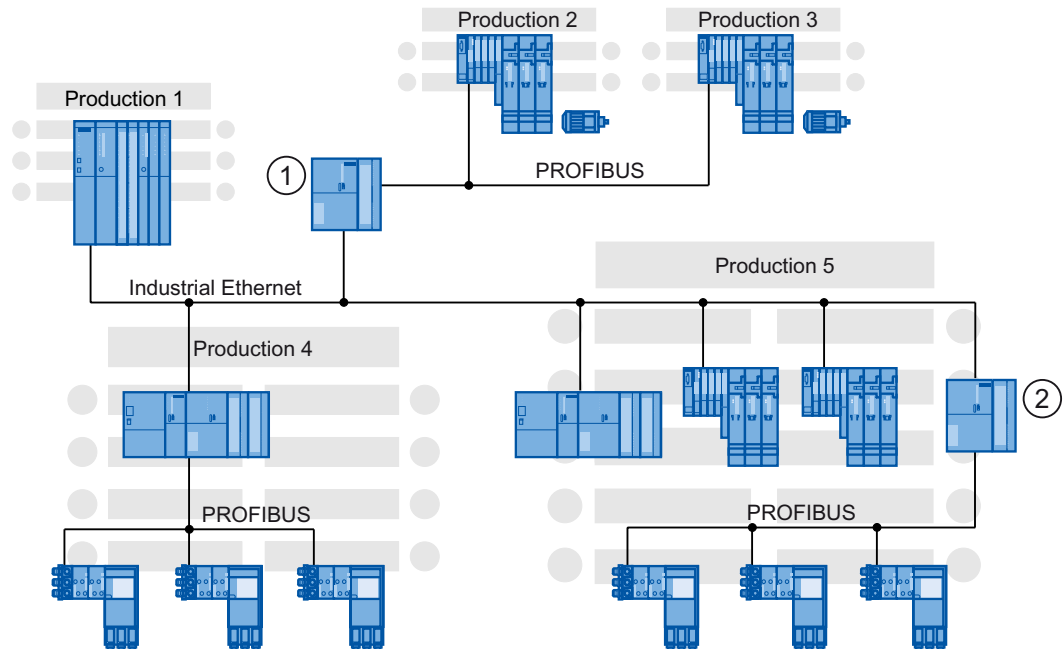
Bild 7-5 Beispiel - Realisierung
