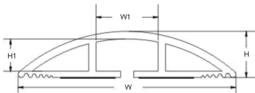
Dimensions : Millimetres
