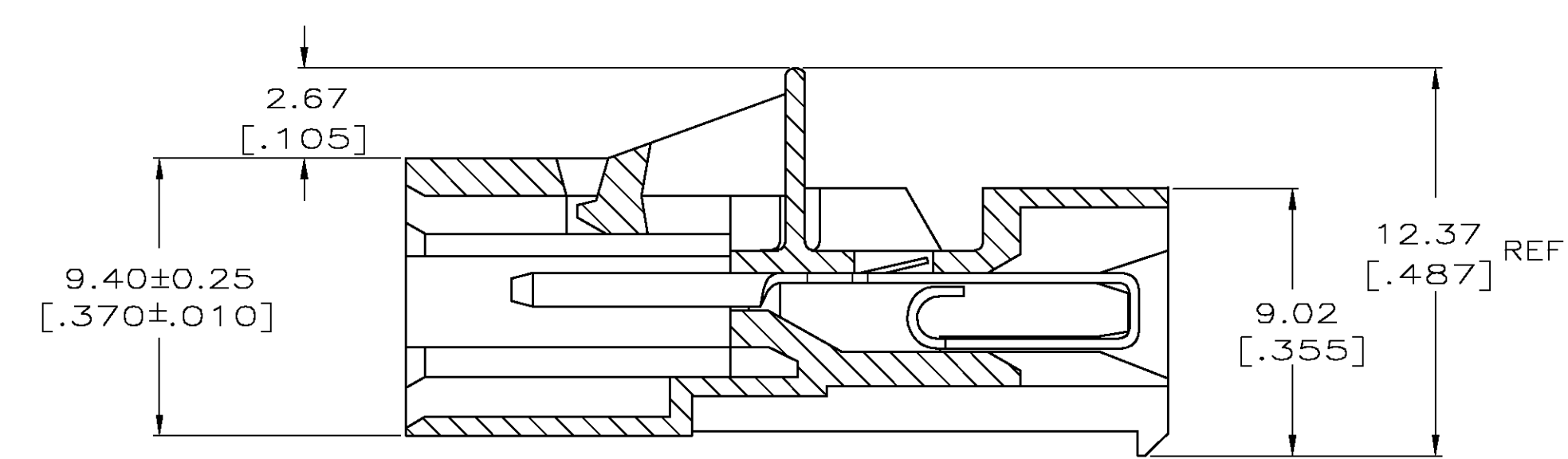
SECTION A-A
