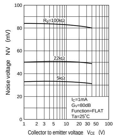
NV - V_{CE}
