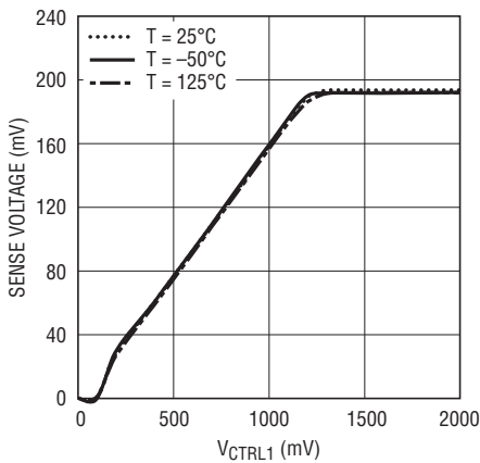
Sense Voltage (V CAP1 - V LED1 ) vs V CTRL1
