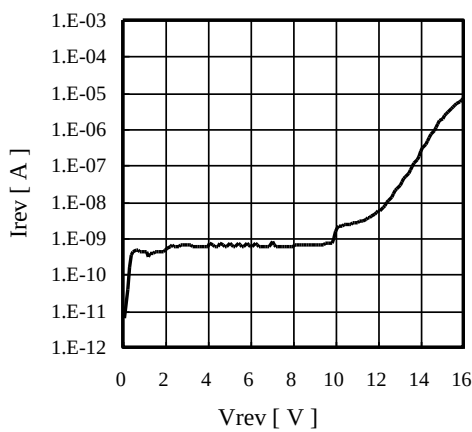
■ I_{\text{Rev}} vs V_{\text{Rev}} (AP1154ADL50)
