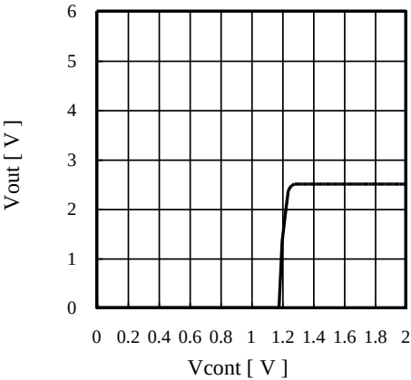
■ V_{out} vs V_{Cont} (AP1154ADL25)
